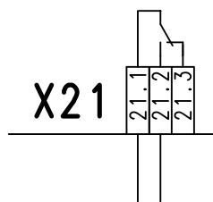
X21 Contact du relais exempt de potentiel
