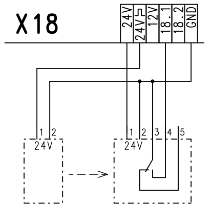
X18 Emetteur Récepteur Cellule photoélectr. unidirect. simple, comme sécurité anti-relevage selon EN 12978
