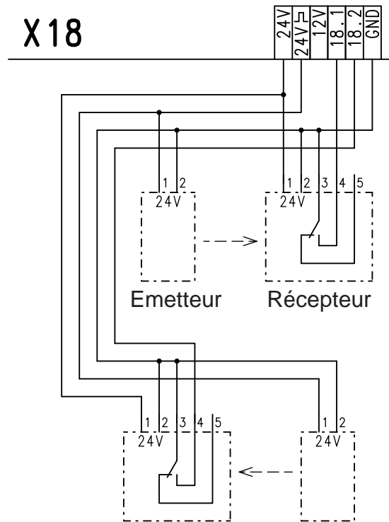
X18 Emetteur Récepteur Récepteur Emetteur Cellule photoélectr. unidirect. double, comme sécurité anti-relevage selon EN 12978
