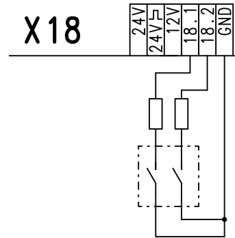
Sortie sécurité anti-relevage externe 1K2 double
