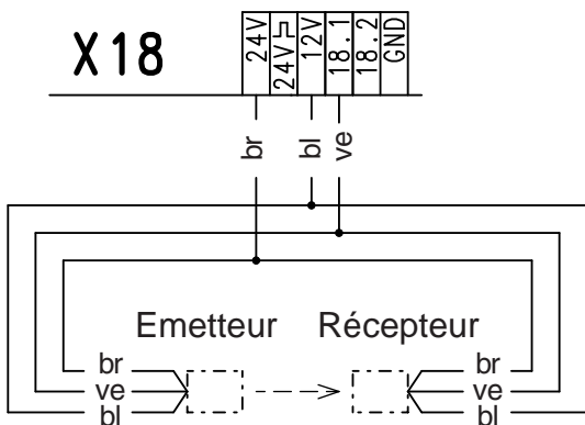
Raytector cellule photo-électrique ou Tige de commande optique comme sécurité anti-relevage simple
