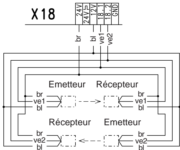
Raytector cellule photo-électrique ou Tige de commande optique comme sécurité anti-relevage double
